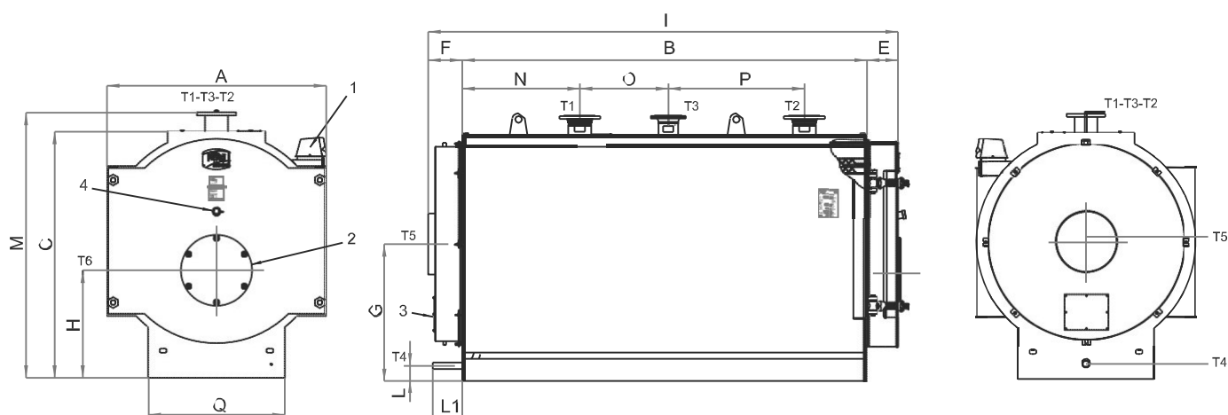
рис. 4 - RSW 2360N+6000N
